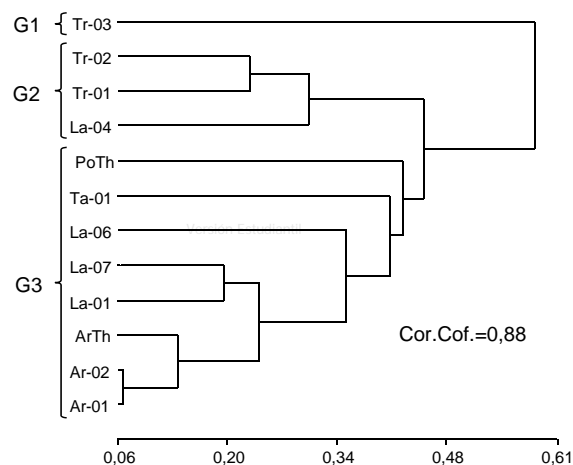
Figura 3. Dendrograma obtenido del algoritmo de UPGMA de los coeficientes de distancia (1-S de Jaccard) con datos de la digestión del rADN-ITS en 12 aislados de Trichoderma spp.
