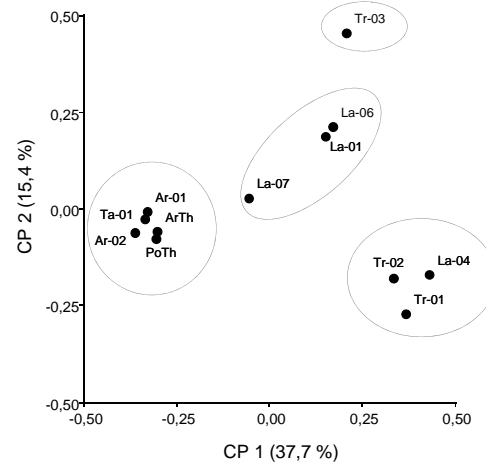
Figura 2. Representación gráfica del análisis de coordenadas principales obtenido de la evaluación de los 12 aislados de Trichoderma spp. utilizando los coeficientes de distancia (1-S de Jaccard) con datos de RAPDs
