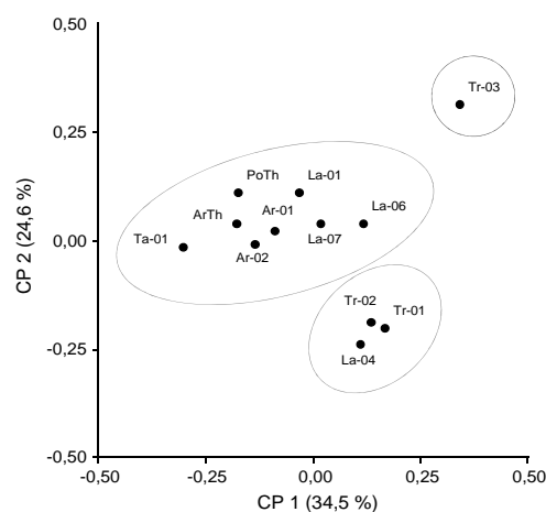
Figura 4. Representación del análisis de coordenadas principales al evaluar los 12 aislamientos de Trichoderma spp. con datos de la digestión del rADN-ITS
