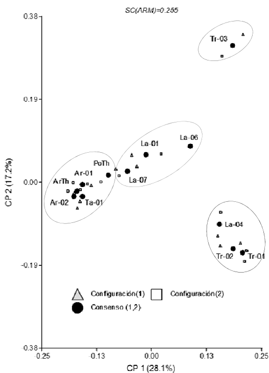
Figura 5. Configuración de consenso del análisis de procrustes generalizado (APG) desde la matriz de datos rADN-ITS y RAPD en 12 aislamientos de Trichoderma spp. Tr-01= T. harzianum , Tr-02= T. harzianum , Tr-03= T. longibrachiatum , La-01= T. pseudokoninngii , La-04= T. atroviride , La-06= T. koningiopsis , La-07= T. koningiopsis , Ar-01= T. harzianum , Ar-02= T. harzianum , Ta-01= T. harzianum , Ar-Th = ( Trichobol ) y Po-Th=( Subiol )
