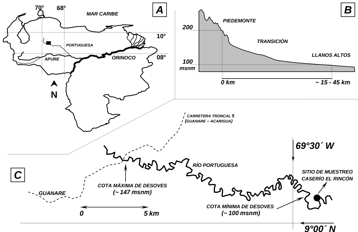
Figura 1. A: Ubicación nacional del área de estudio. B: Perfil, anchura y desniveles aproximados de la zona de transición geomorfológica entre los llanos altos y el piedemonte del río Portuguesa, (escala vertical ampliada) C: Plano de la zona de transición del río Portuguesa mostrando las cotas mínimas y máximas estimadas para los desoves
